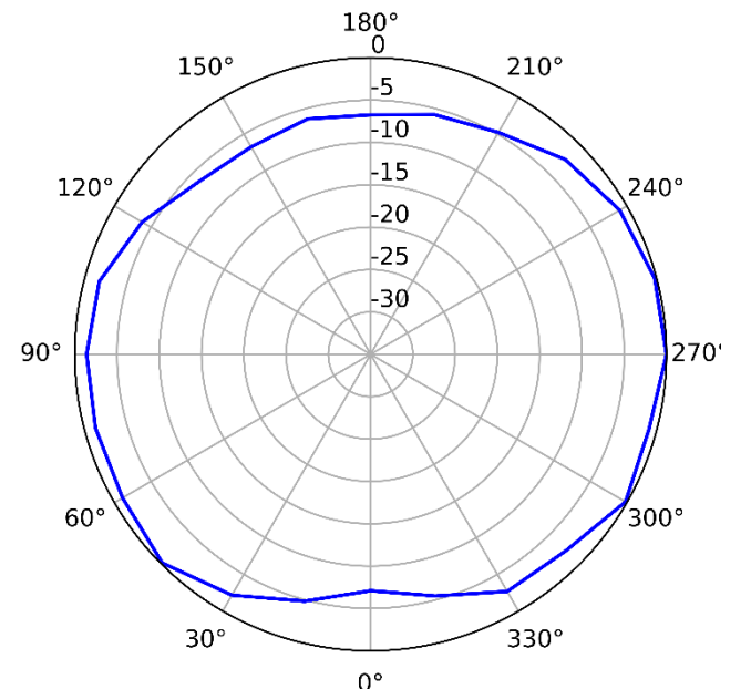
5 GHz (vertical)
