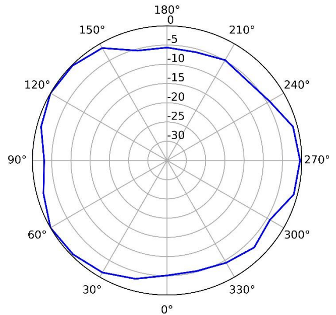
2.4 GHz (vertical)
